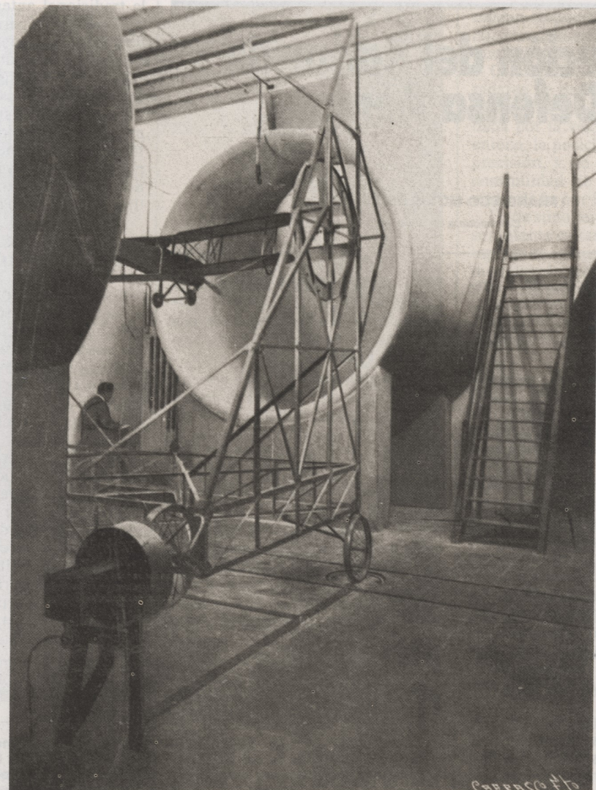
Balanza aerodinámica universal.
